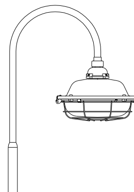
スタンド形
