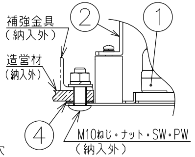
器具取付詳細図
