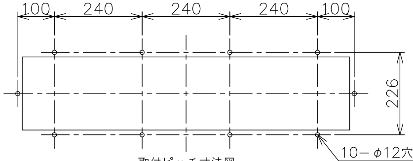
取付ピッチ寸法図
