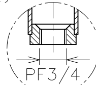
A部詳細
