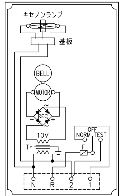
結線図
