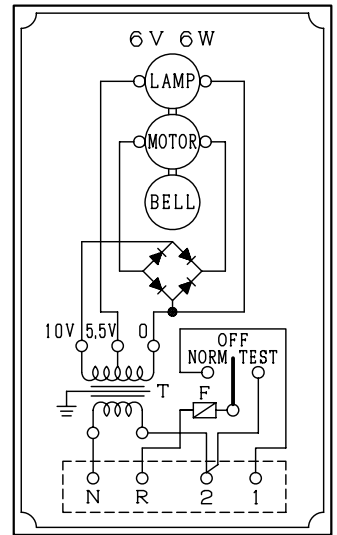
結線図
