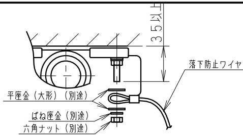
落下防止ワイヤの取付要領図
