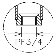
A部詳細
