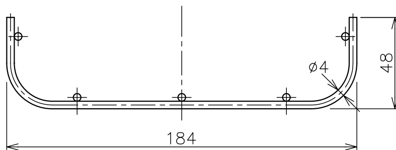
A 視 図 (S=1/2)
