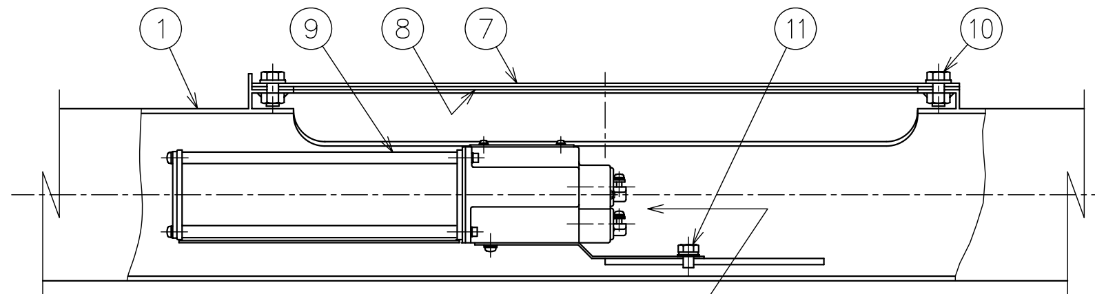
安定器収納部詳細 1/5 パッキン式引込方式 ケーブル仕上り外径：2-ø13.5~ø18
