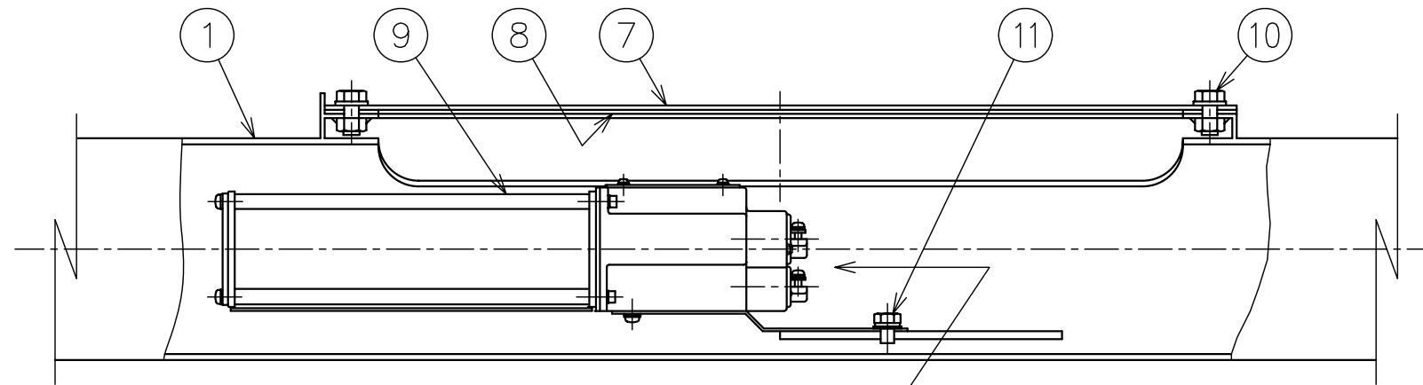
安定器収納部詳細 1/5
