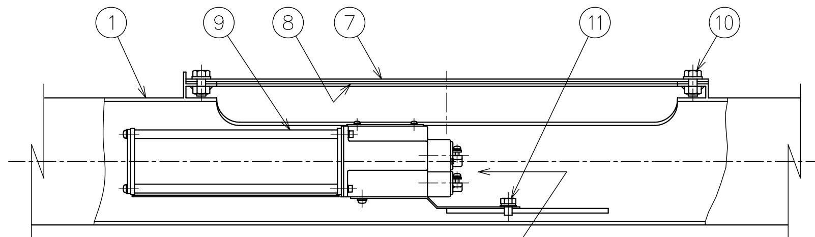
安定器収納部詳細 1/5
