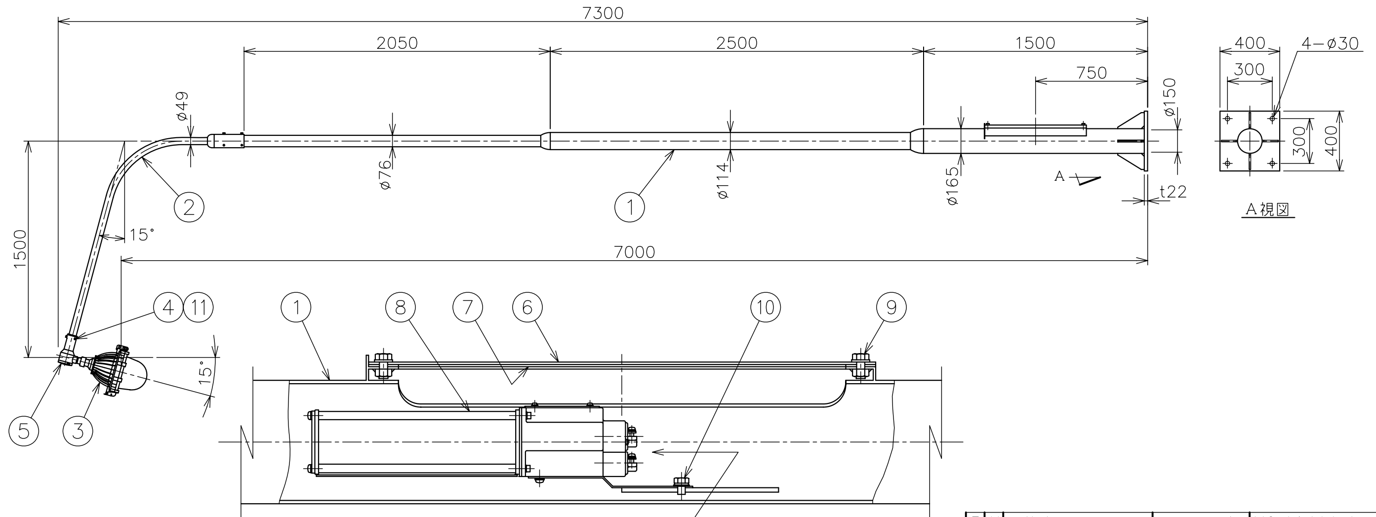
安定器収納部詳細 1/5
