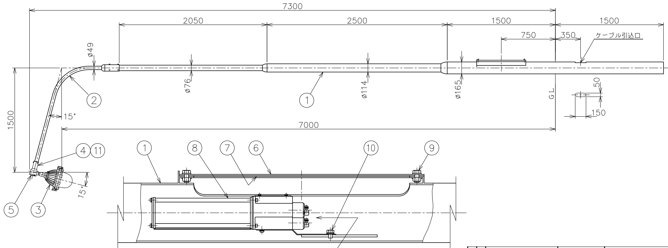
安定器収納部詳細 1/5
